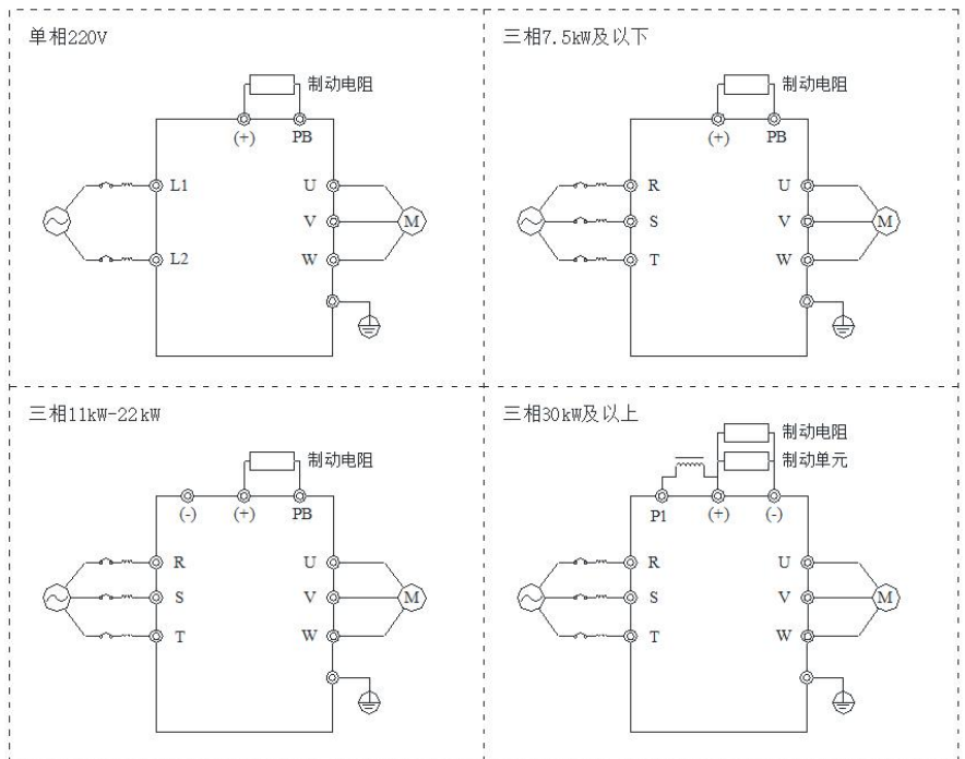
图 3-1 变频器主回路接线方式
