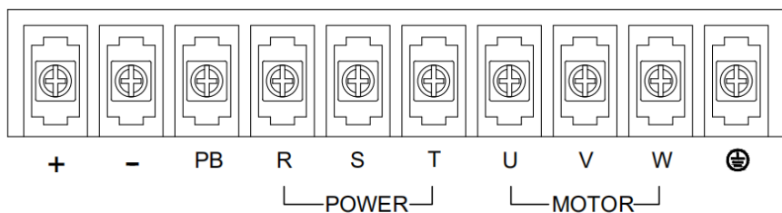
18~22KW标准品主回路端子
