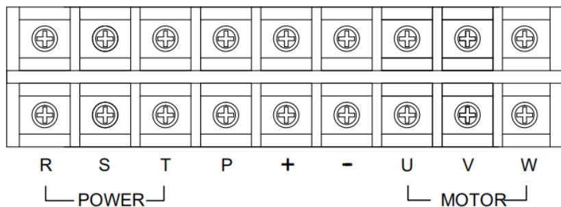
90~110KW标准品主回路端子
