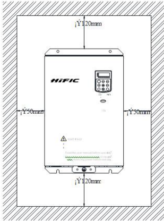
单台变频器安装示意图
