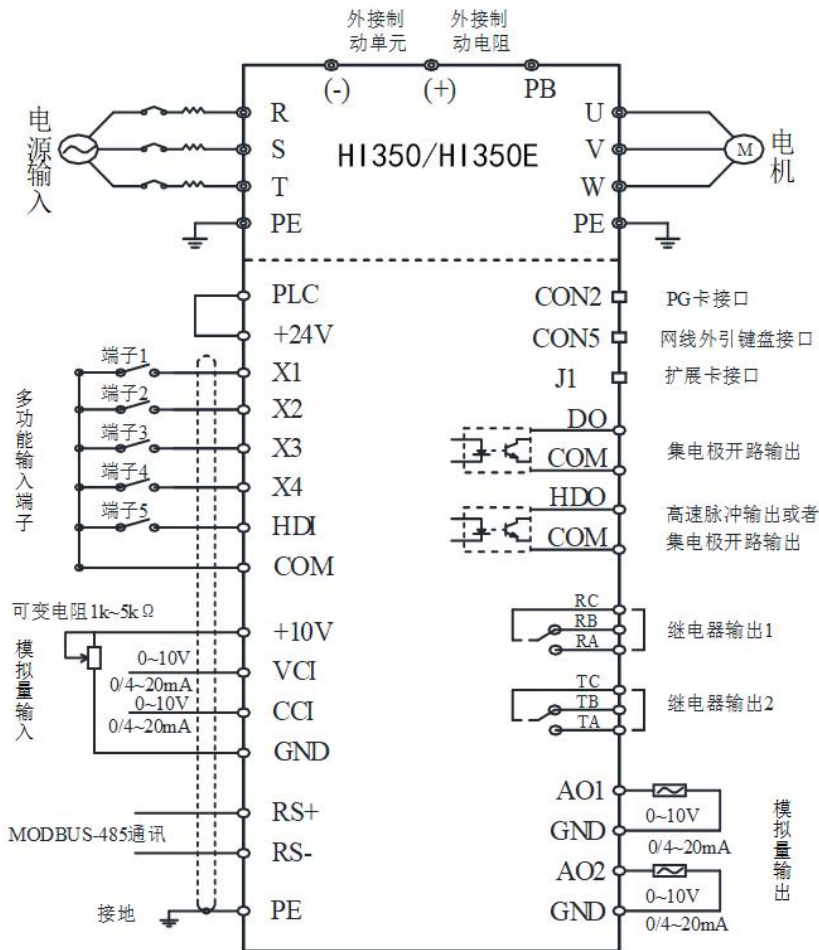
图3-2 控制回路连接方式
