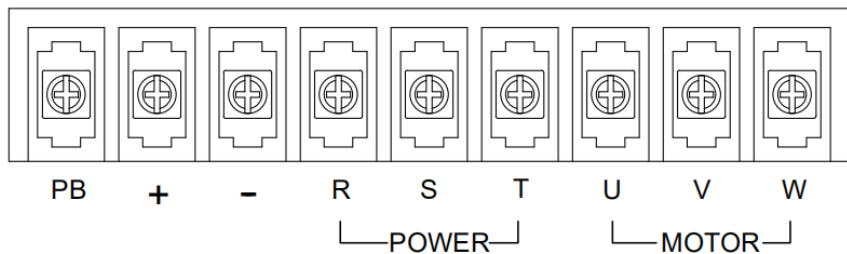
0.75~15KW标准品主回路端子
