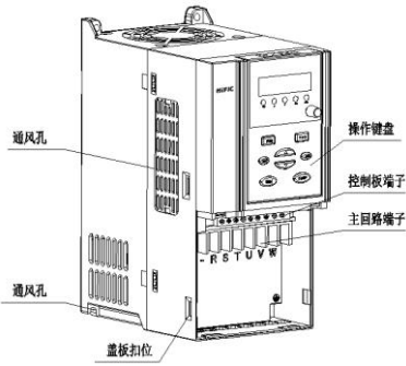
图2-2 HI350 系列变频器塑胶结构外型图
