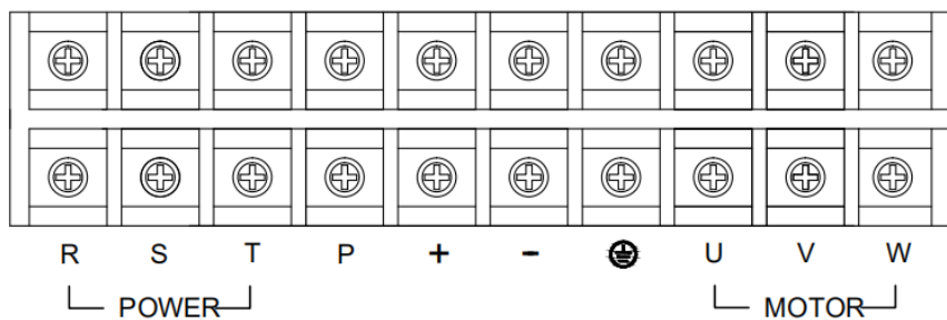
132~160KW标准品主回路端子
