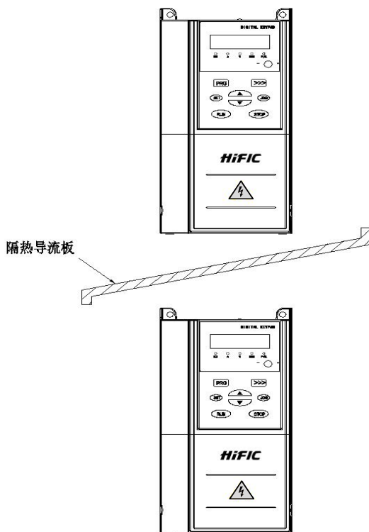
图2-7 多台变频器安装及通风设置
