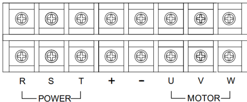
45~75KW标准品主回路端子
