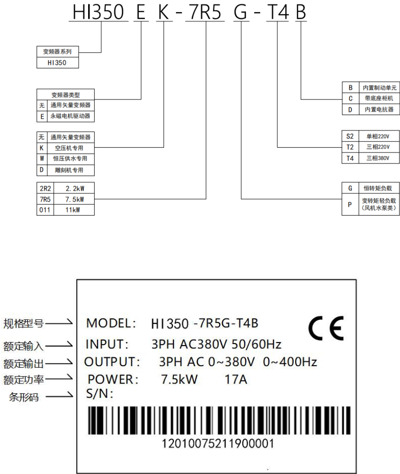
图 2-1 产品命名与铭牌标识
