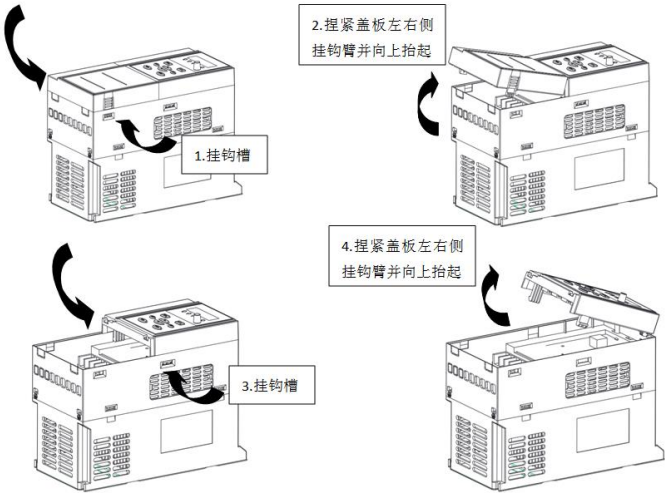
图 2-3 塑胶外壳盖板拆卸图
