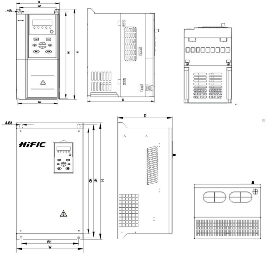
图2-4 外形及尺寸
